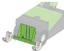
Adapter voor winkelwagens (90°) Artikel Nr OPT0324
