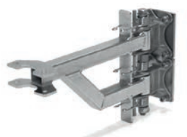
Basisdeel HD-haak 90° (verhoogd) Artikel Nr H7080
